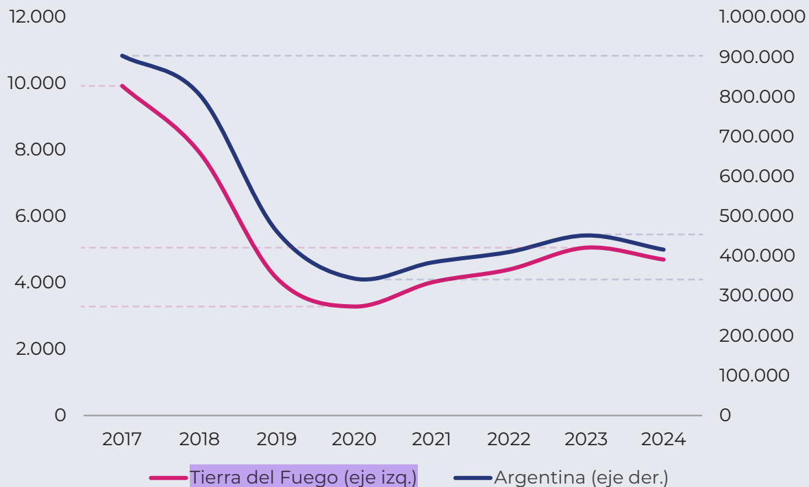
Fuente 12. Patentamientos de automóviles acumulados, 2017-2024. En unidades.
