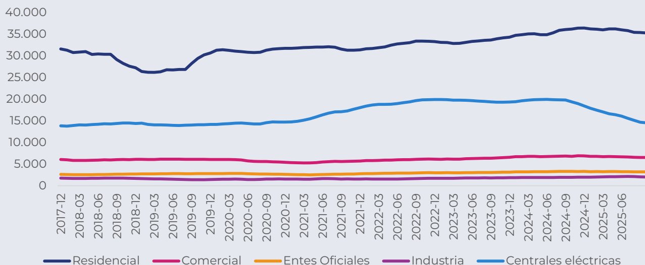
Figura 4. Demanda de gas natural de red, Tierra del Fuego, 2017-2025. En miles de m 3 , media 12 meses.
